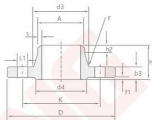
DIN 2633
